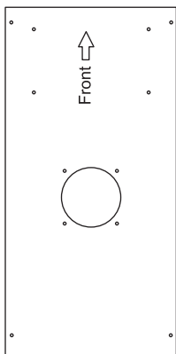
2006-ACIV-03 天板
