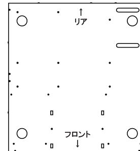
底面板 2007-ACVI-04
