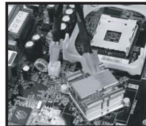
電源側 ATX12V (4ピンのみ使用)
