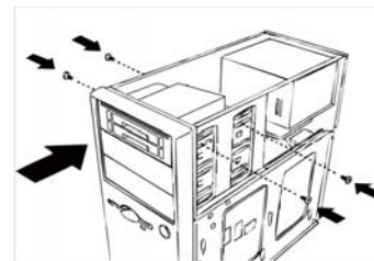
両サイドからネジ留めて固定する
