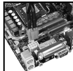
電源側 EPS12V(4+4ピン)
