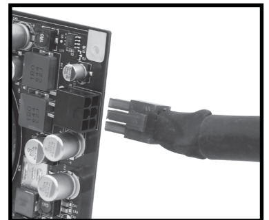
写真はPCI-E(6ピン)仕様のグラフィックスカードのものになります。
