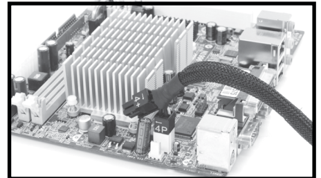
ATX12V(4ピンのみ使用)
