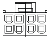
電源側 EPS12V(4+4ピン)
