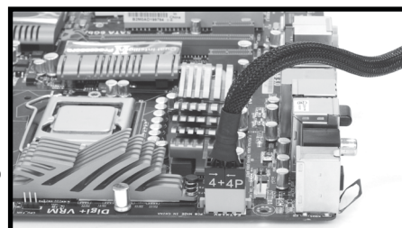
電源側 EPS12V(4+4ピン)
