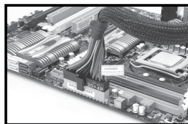
マザーボード側 ATXメインコネクタ
