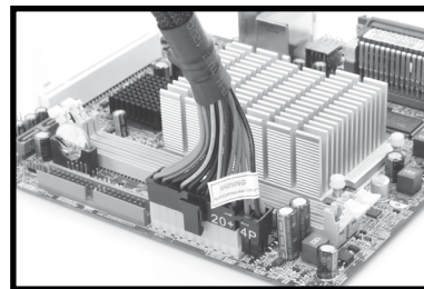
電源側 ATXメイン(20ピンのみ使用)
