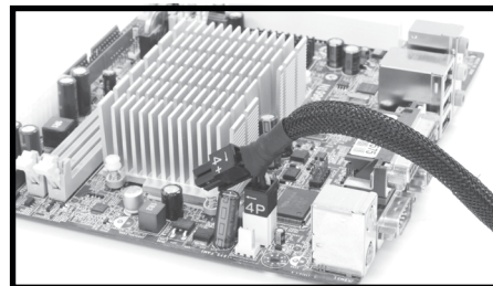
電源側 ATX12V (4ピンのみ使用)
