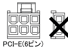
PCI-E(6ピン)
